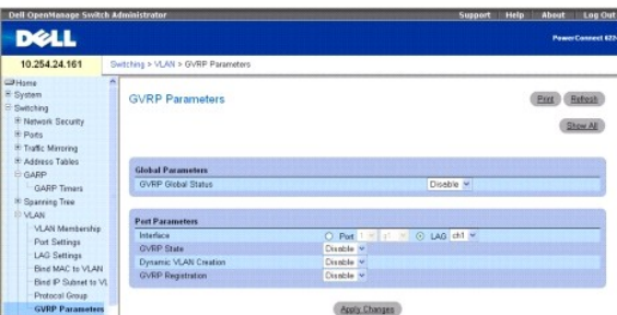
Ilustración 8-62. Parámetros globales de GVRP
